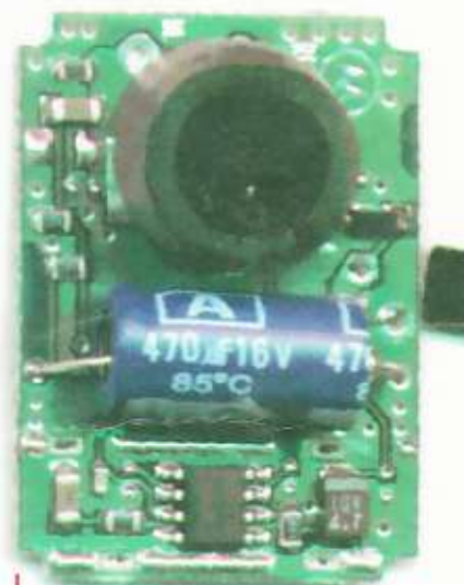
Van boven naar beneden: de microfoon, de elco in het midden is voor de ontkoppeling van de voedingsspanning en het IC onderaan is de versterker.
